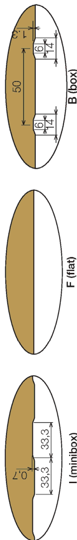
Deckschichtvarianten (Innenseite)
