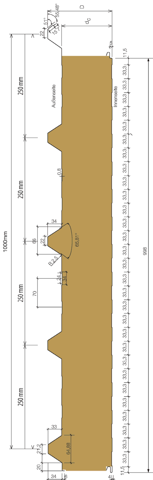
Deckschichtvariante (Außenseite) T (trapez)
