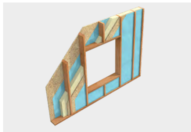
Voorbeeld van een HSB-gevelelement
