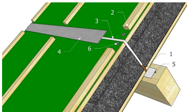
Figuur 6 - Detail horizontale naden
