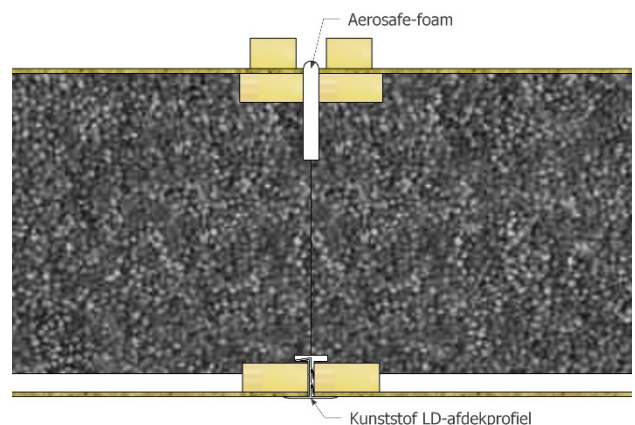
Figuur 5 - Detail Aerosafe-foam en Kunststof LD-afdekprofiel
